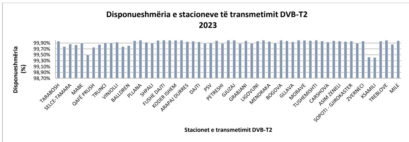
Grafiku 2. 3. Disponueshmëria e Stacioneve (%)
